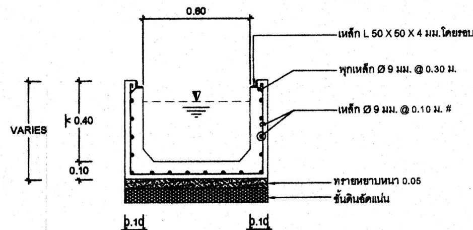
ขยายวางระบายน้ำ 2 มาตรฐาน 1:20
