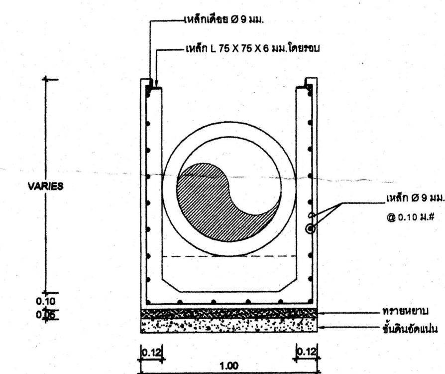
แบบขยายป้อมกั้น MH1 มาตรฐาน 1:20
