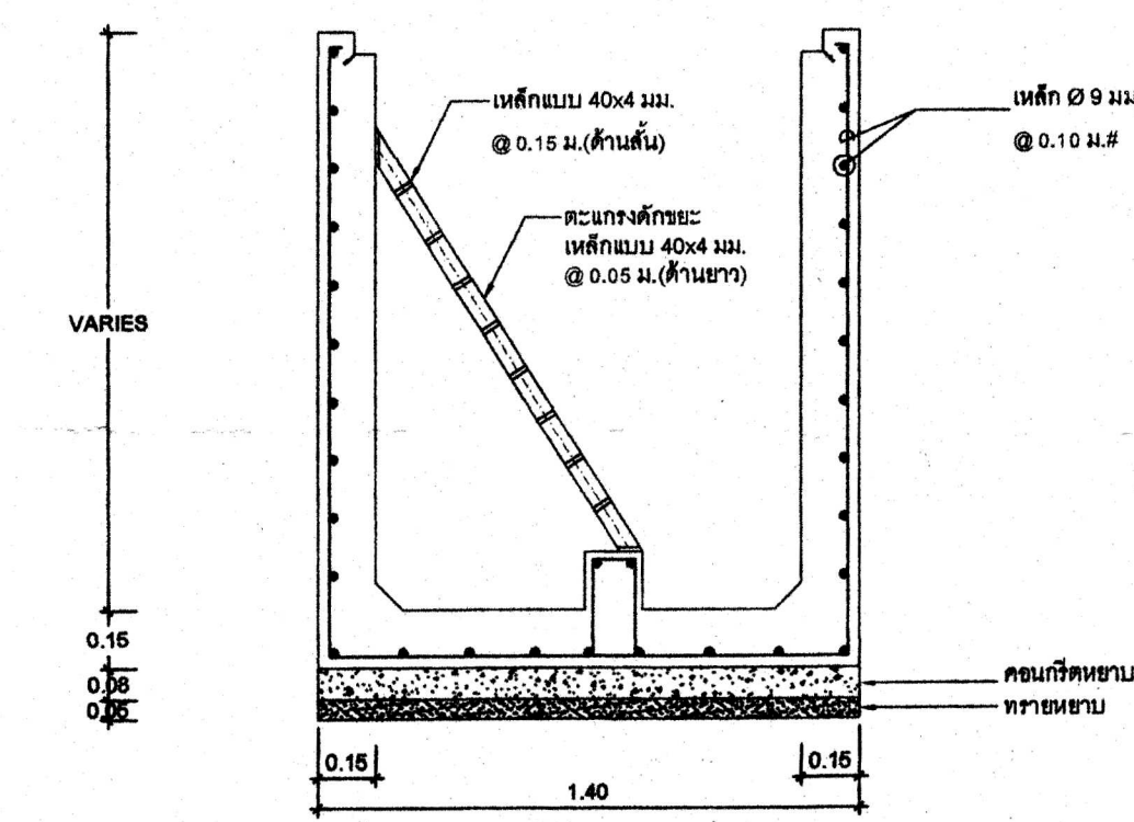
แบบขยายป้อมกั้น MH2 มาตรฐาน 1:20
