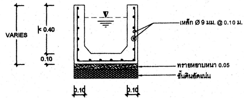
ขยายวางระบายน้ำ 1 มาตรฐาน 1:20
