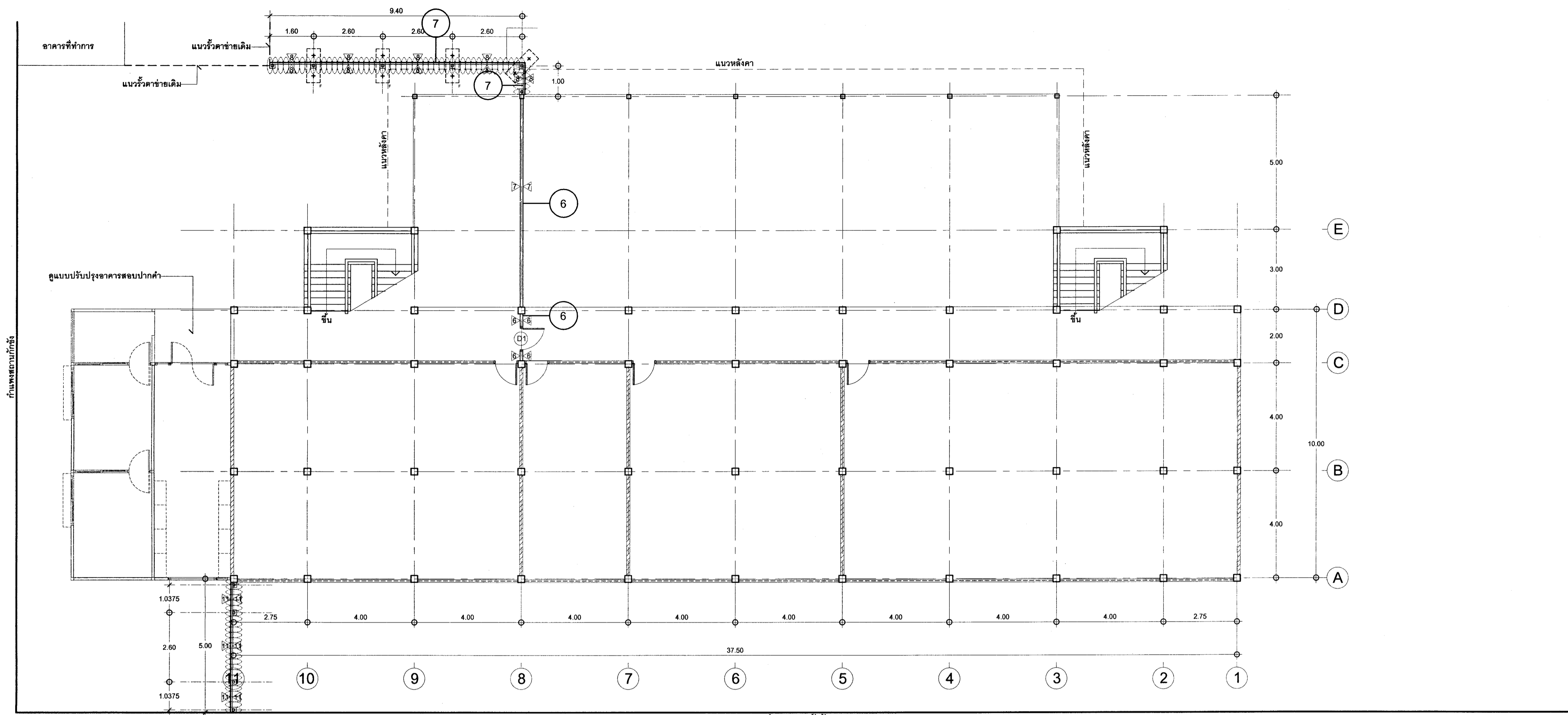
แปลนพื้นเรือนนอนชายชั้นล่างปรับปรุง หมายเหตุ - ระบกก่อสร้างในแบบแปลนอาคาร เป็นระบกก่อสร้างโดยประมาณ ให้ผู้รับจ้างดำเนินการตรวจสอบหน้างานจริงอีกครั้ง หากมีความคลาดเคลื่อนให้ผู้รับจ้างจัดทำ SHOP DRAWING เสนอผู้ควบคุมงานและคณะกรรมการตรวจการจ้าง พิจารณาอนุมัติก่อนดำเนินการ โดยจะคิดเป็นมูลค่างานเพิ่มไม่ได้
