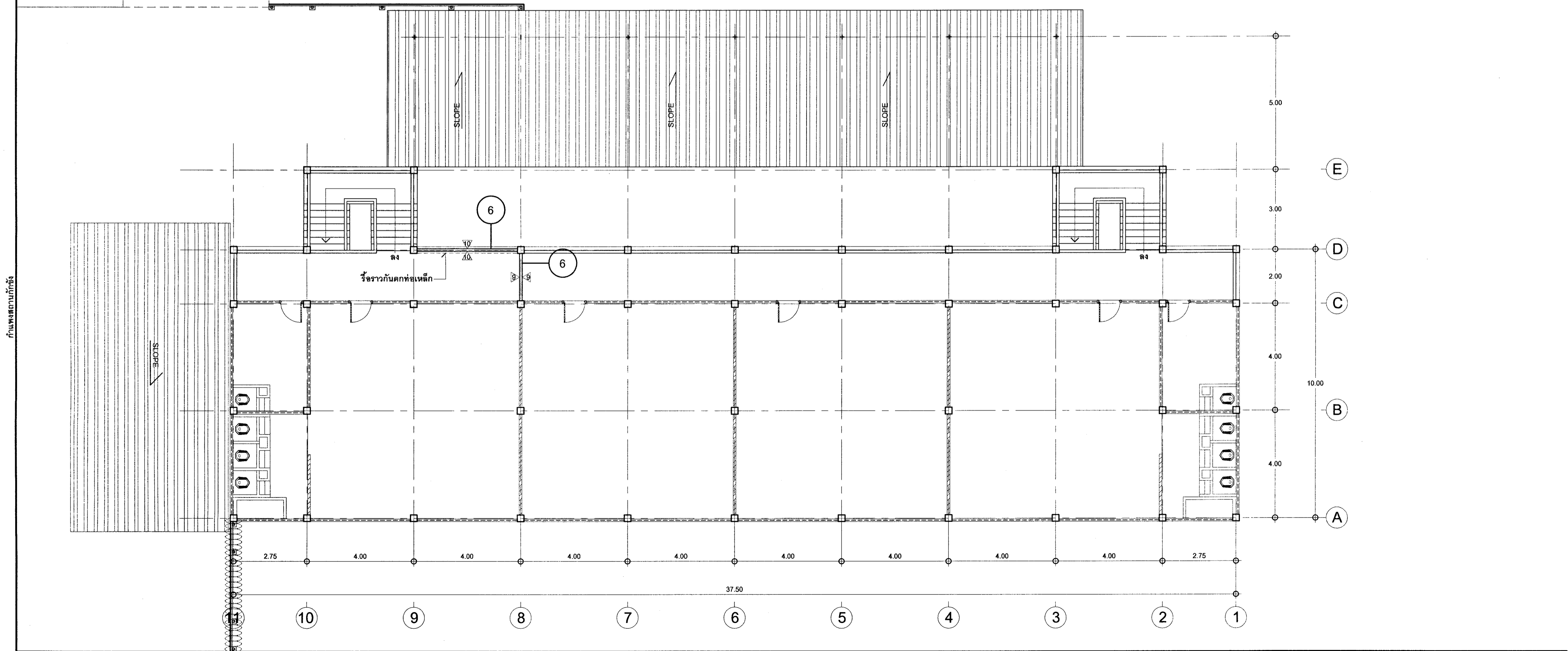
แปลนพื้นเรือนนอนชายชั้นบนปรับปรุง
